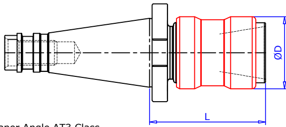
CHUCK TYPE SCDTC../MT.
